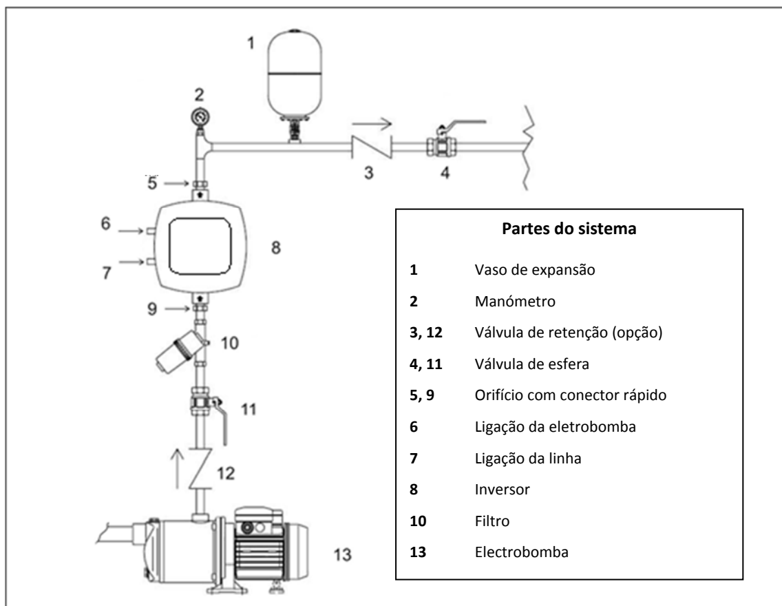
Figura 1: Instalação hidráulica
