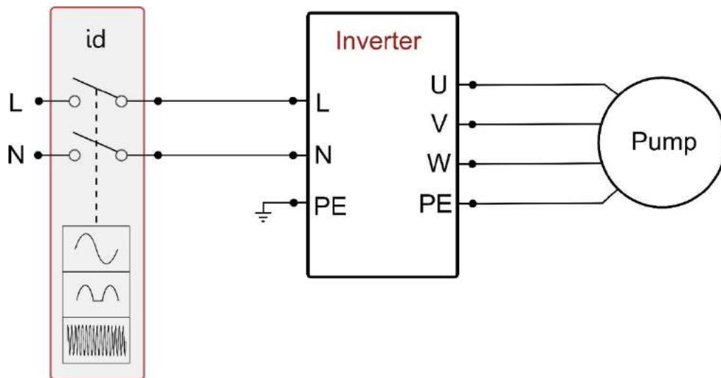
Figure 2a: Exemple d'installation avec alimentation monophasée
