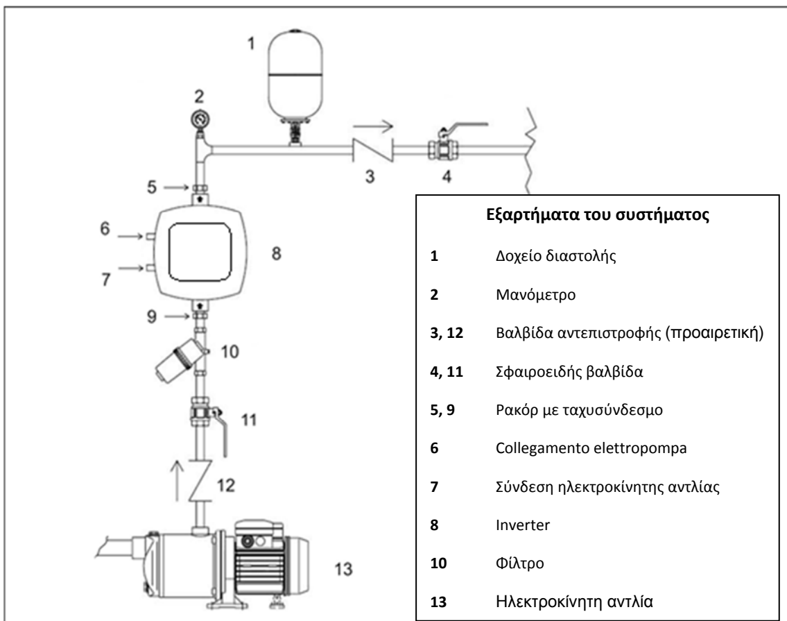
Σχήμα 1: Υδραυλική εγκατάσταση
