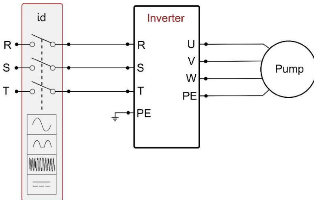
Figure 3b: Exemple d'installation avec alimentation triphasée
